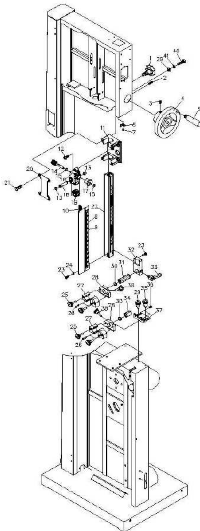
Чертеж №4 Узел верхних и нижних направляющих полотна
