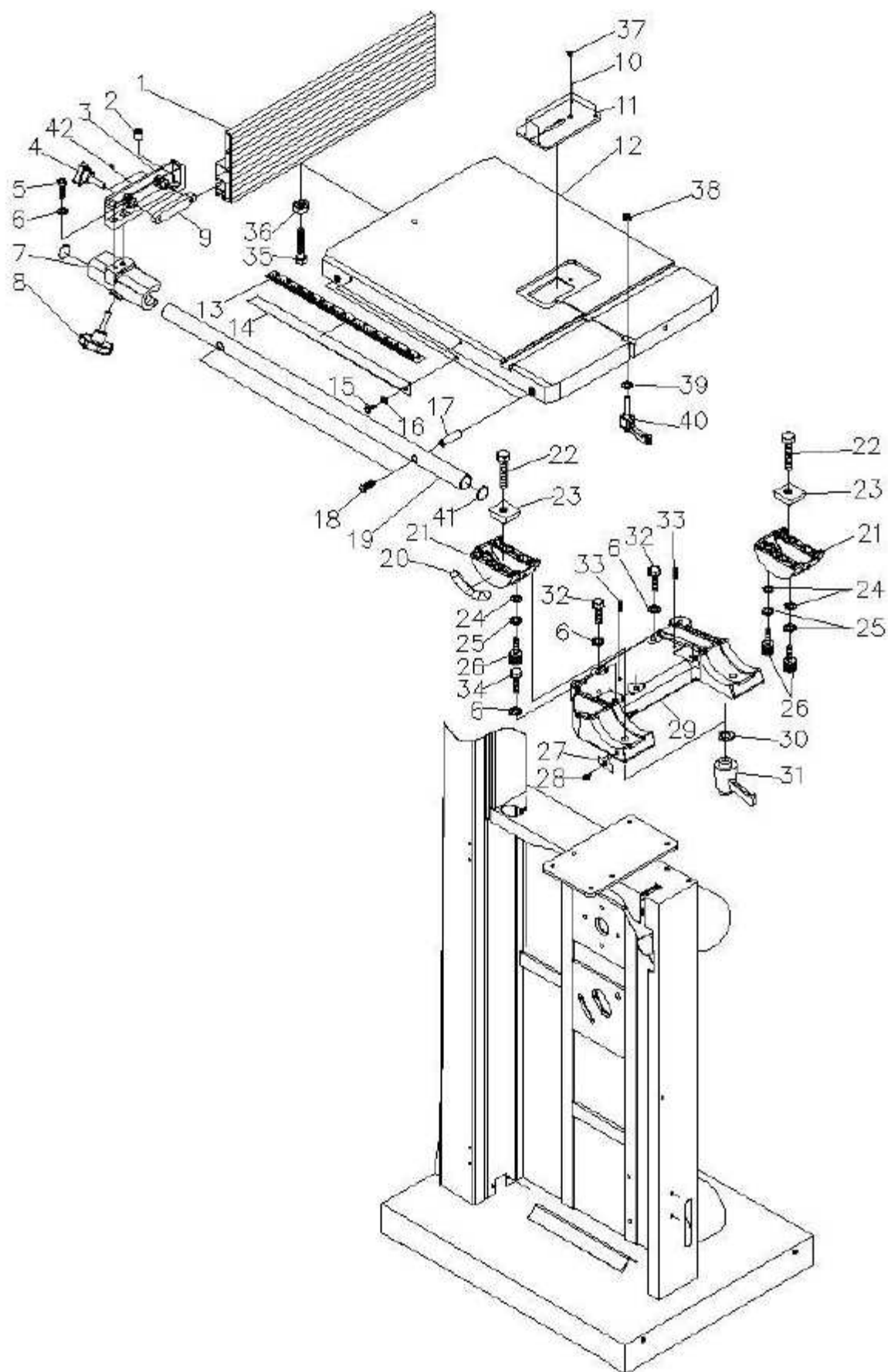
Чертеж № 3 Узел стола и параллельного упора
